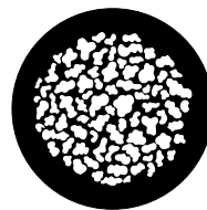
外径: Ø32.0 图案: Ø26 厚度: 1.1mm 位置: 5
